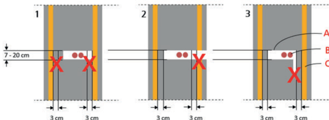
Abbildung 14: 3 Fehler, die bei der Installation vermieden werden müssen!
