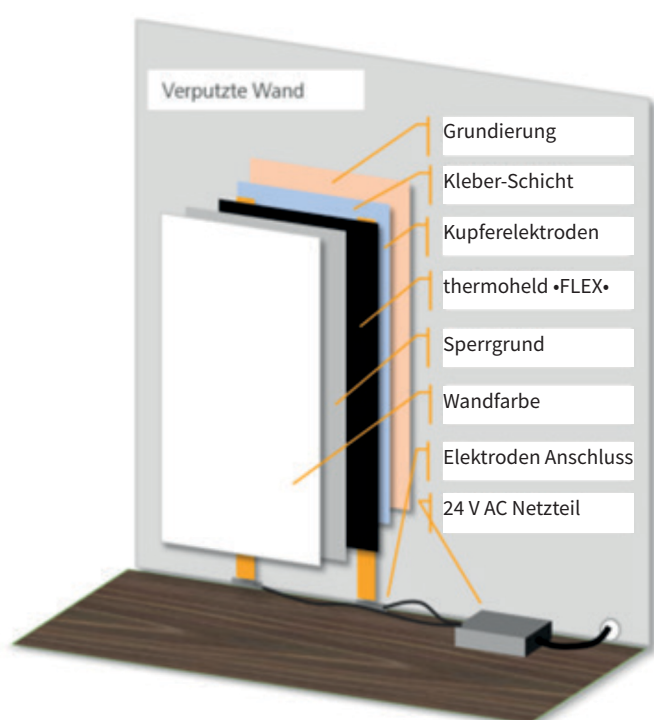
Abbildung 3: Typischer Schichtaufbau der thermoheld •FLEX• Heizfläche am Beispiel einer verputzten Wand
