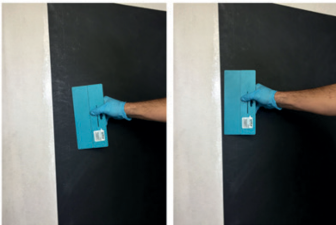
Abbildung 6: Ausstreichen der Blasen von innen nach außen
