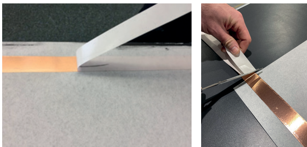
Abbildung 4: Abziehen der weißen Schutzfolie von den Elektrodenbändern
