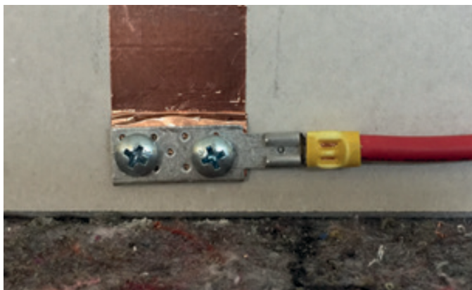
Abbildung 11: Elektrodenkontaktierung zur sicheren Verbindung zwischen der thermoheld •FLEX• Heizschicht und der Spannungsversorgung
