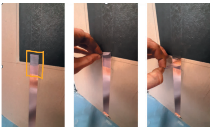
Abbildung 9: Abziehen des farbigen Sicherungsbandes (im Bild gelb markiert), beginnend über dem schwarzen Heizvlies
