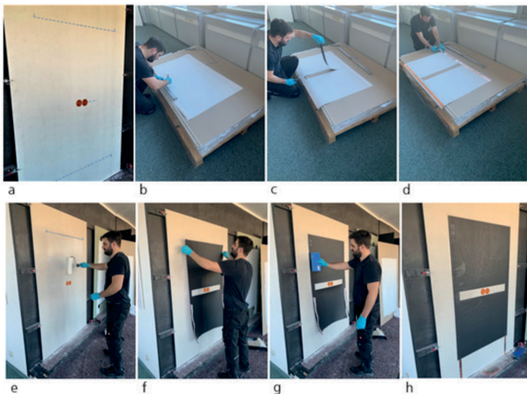
Abbildung 13: Installation der thermoheld •FLEX• Heizfläche mit Aussparung
