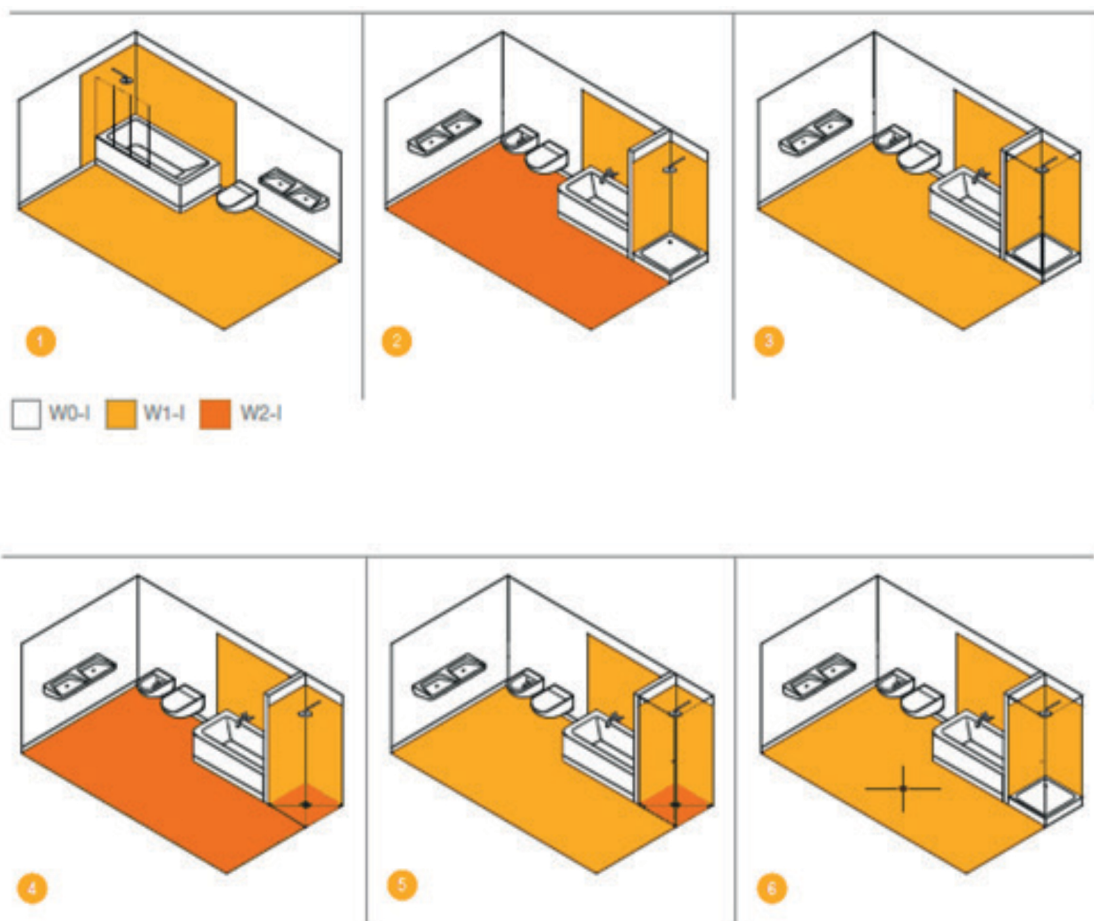
Abbildung 1: Beispiele für die Wassereinwirkungsklassen nach DIN 18534 in verschiedenen Badsituationen. Die zu berücksichtigenden Flächen, die abgedichtet werden müssen, wurden gelb Einwirkungsklasse W1-I und orange Einwirkungsklasse W2-I markiert.
