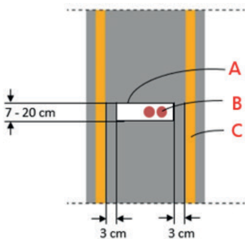
Abbildung 12: thermoheld •FLEX• Heizfläche mit Aussparung A um eine Steckdose B in Form eines Rechtecks, Höhe des Rechtecks: 7 – 20 cm, Breite: definiert durch jeweils 3 cm Abstand zur Innenkante der Elektrode C
