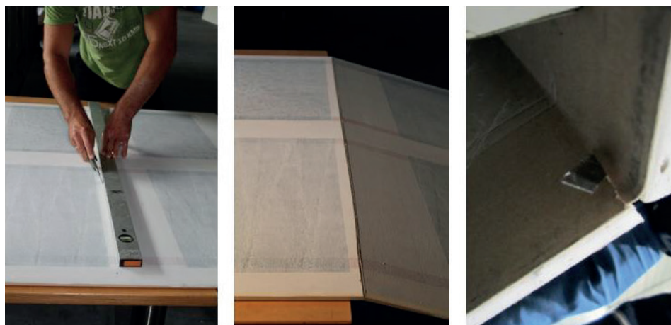
Abbildung 7: Zum Teilen der thermoheld •WAND• erst sauber anreißen, dann Platte brechen und zum Schluss rückseitigen Karton durchtrennen
