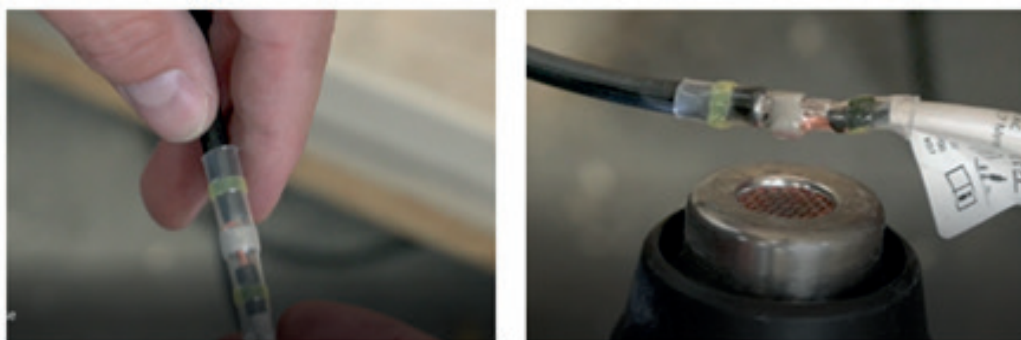
Abbildung 24: Verlängern der Zuleitungen mithilfe der beigelegten Lötverbinder
